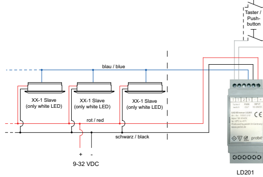
Profil 2-Kanal / profile 2-channel:
